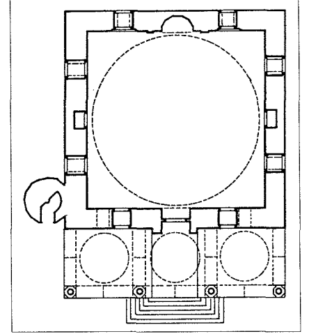
Firuz Ağa Camii'nin planı
